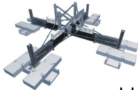
Neigbare Fundamentfüße/CP-Gestänge
